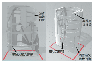
曾侯乙编钟的三维设计模型。
